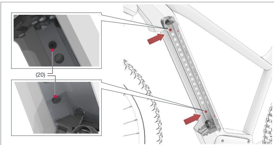
H. Vibrationsdämpfer
